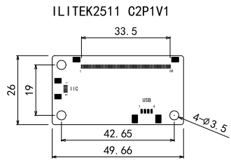
CONTROLLER SC 2:1
